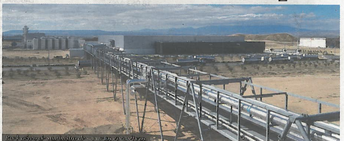
Rack aéreo de suministro de servicios energéticos.
