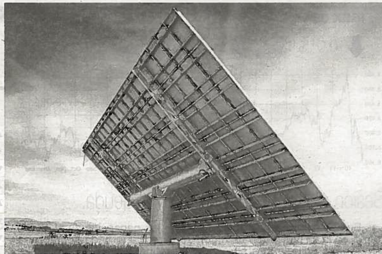
Imagen del seguidor solar fabricado por Clavijo. FOTO: D.N.
